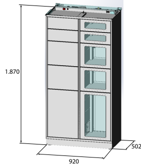
Locker puerta S, M y L
